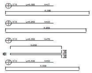
철근재량표
